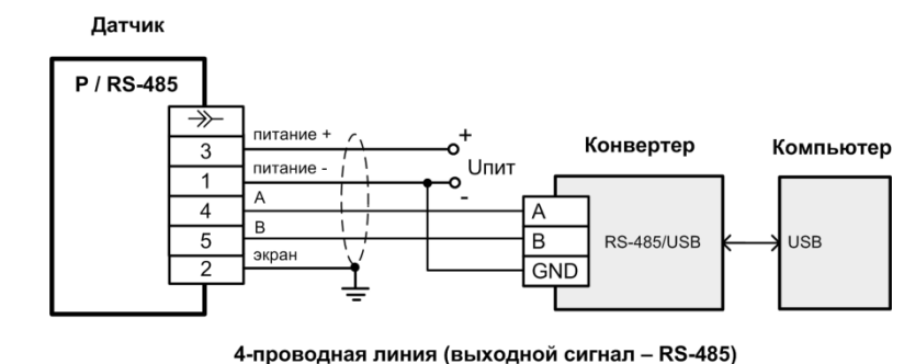
Рисунок 1 – Пример схемы подключения цифрового выхода RS-485 для разъема Binder
