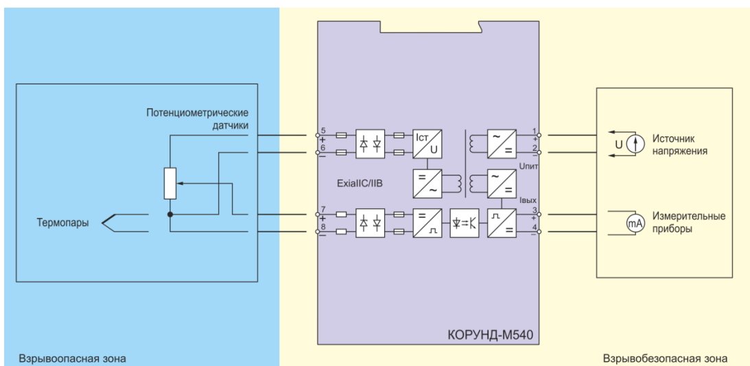
Рис. 2.2. Подключение термопар и потенциметрических датчиков
