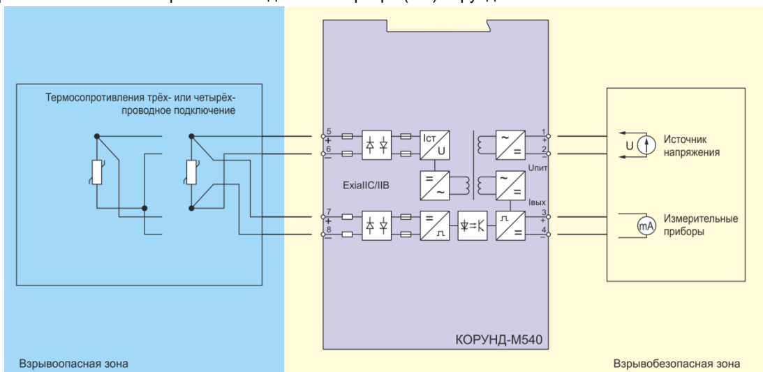
Рис. 2.1. Подключение термосопротивлений
