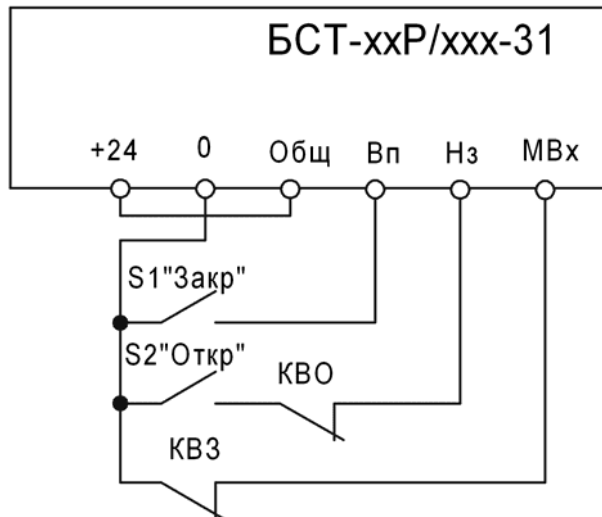
S1, S2 – управляющие выключатели КВ3, КВО – концевые выключатели а) пример №1
