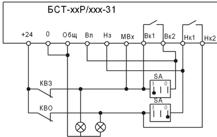
SA – переключатель без фиксации КВ3, КВО – концевые выключатели б) пример №2
