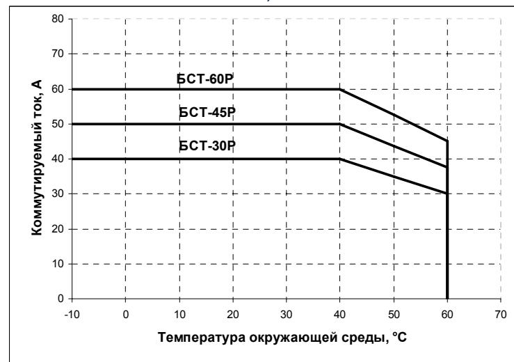
Рисунок 12 – Зависимость коммутируемого тока от температуры окружающей среды:
