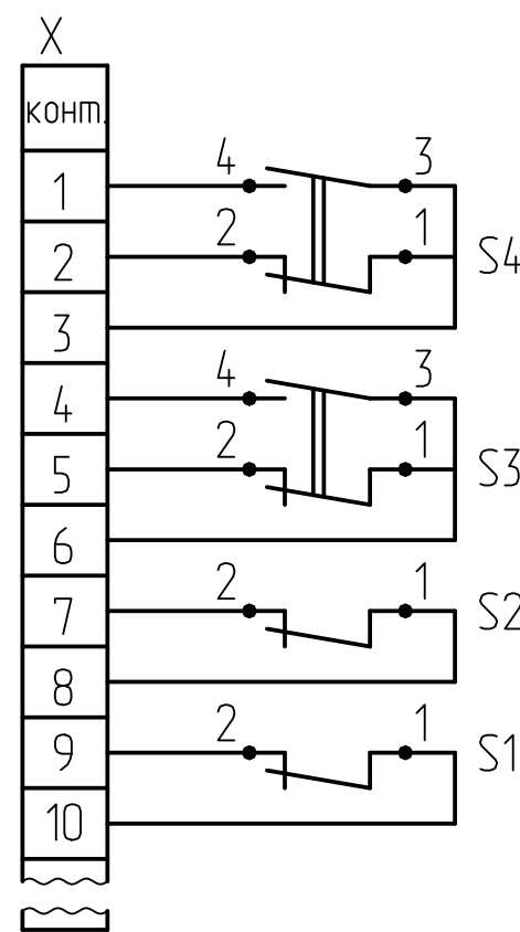
Рисунок В.3 -Схема электрическая принципиальная блока БСПТ-ИВТ6
