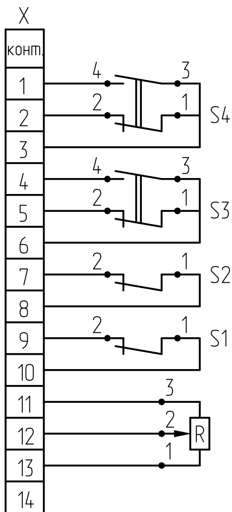
Рисунок В.2 -Схема электрическая принципиальная блока БСПР-ИВТ6
