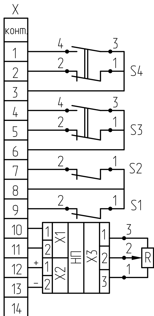
Рисунок В.1 -Схема электрическая принципиальная блока БСПТ-ИВТ6
