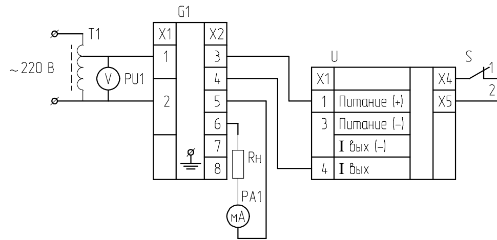
Рисунок А.1 – Схема проверки при двухпроводном соединении блока БД – 10АМ к блоку питания.
