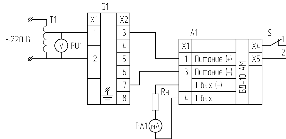
Рисунок А.4 – Схема проверки при четырехпроводном соединении блока БД – 10АМ к блоку питания
