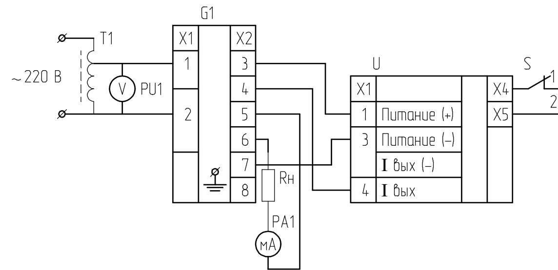
Рисунок А.3 – Схема проверки при трехпроводном соединении блока БД – 10АМ к блоку питания
