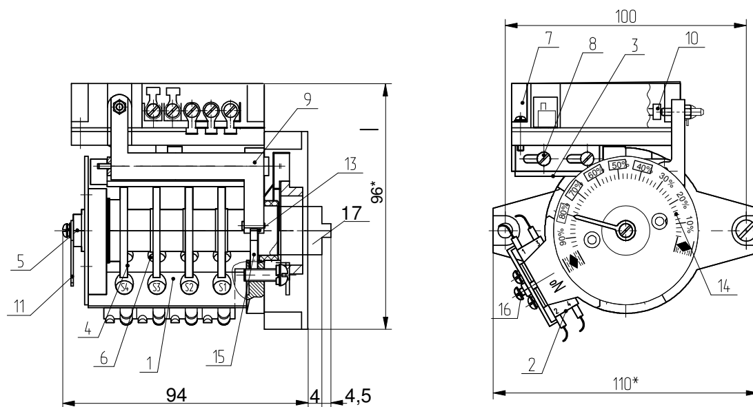
Рисунок Б.1- Общий вид, габаритные и установочные размеры блока БД-10АМК
