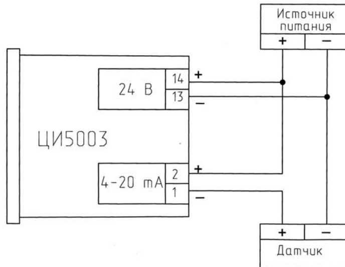
Рисунок Б.1- Схема внешних соединений прибора ЦИ5003Б и датчика с двухпроводной линией связи при раздельном питании.
