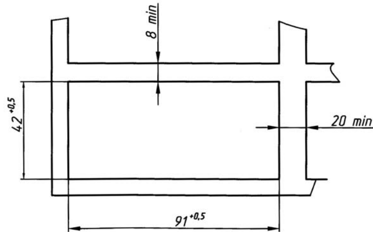
Рисунок А.1- Габаритные размеры прибора ЦИ5003.
