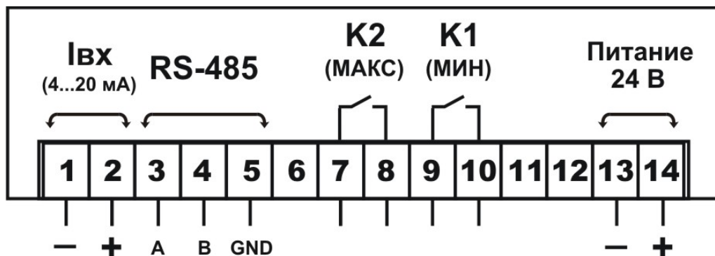
Рисунок Б.5- Расположение выводов клеммной колодки прибора
