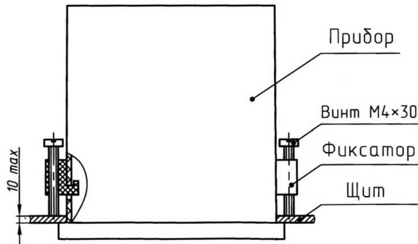
Рисунок А.3- Установка прибора в щите.
