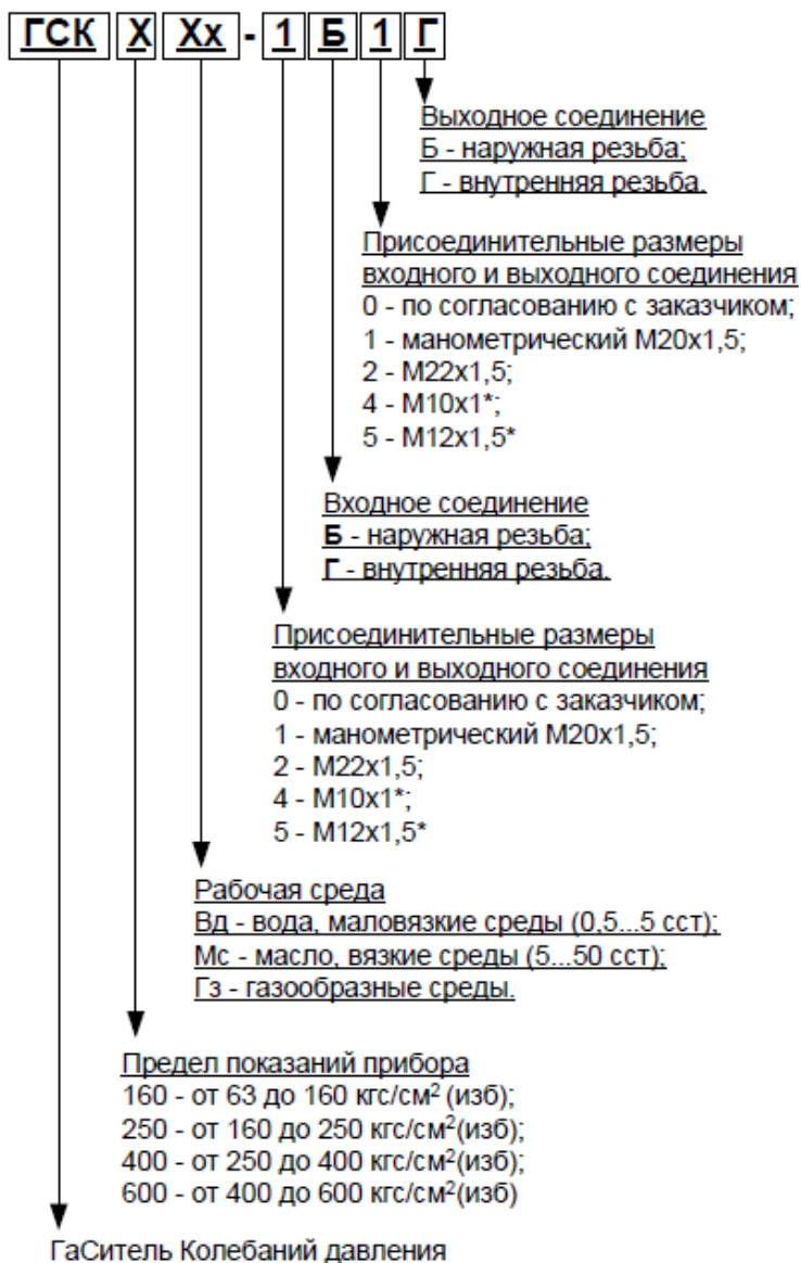
Рисунок 1.1 – Условное обозначение гасителей колебаний давления 1.2 Технические характеристики
