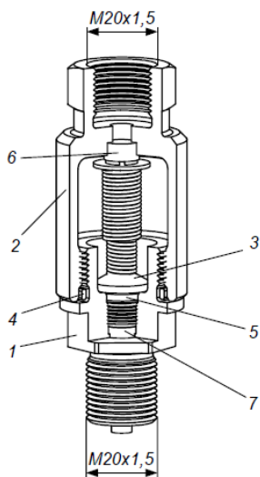
Рисунок 1.2 – Устройство гасителя колебаний давления ГСК250Мс-1Б1Г: 1 – корпус; 2 – крышка; 3 – демпфирующая вставка; 4, 5 – уплотнительное кольцо; 6, 7 – фильтр.
