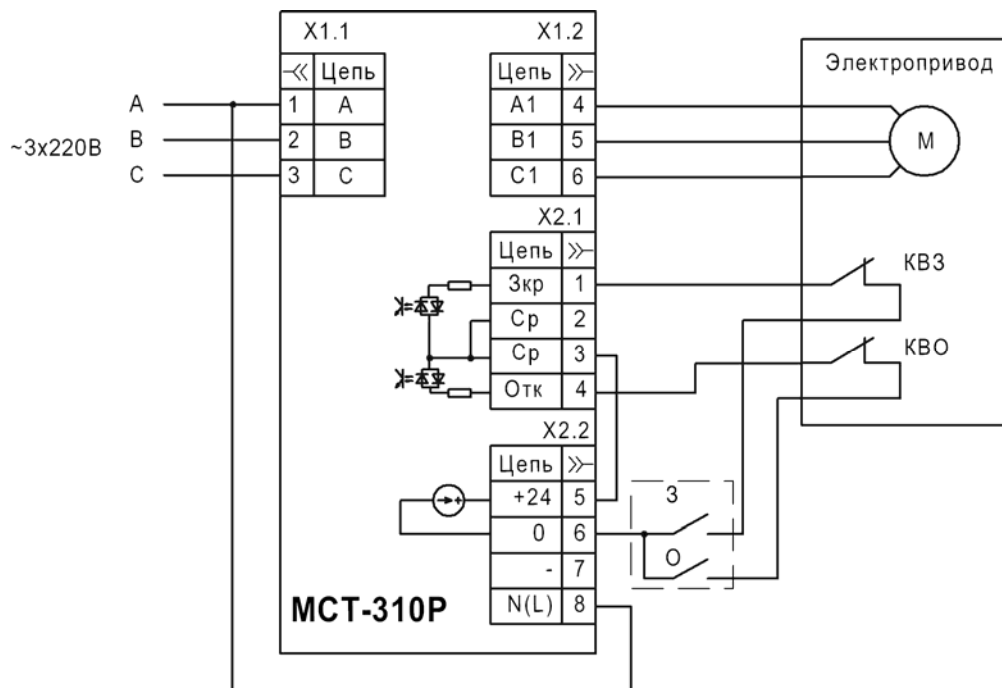
Рисунок 2 –Пример схемы подключения а) для сети 3x380В б) для сети 3x220В
