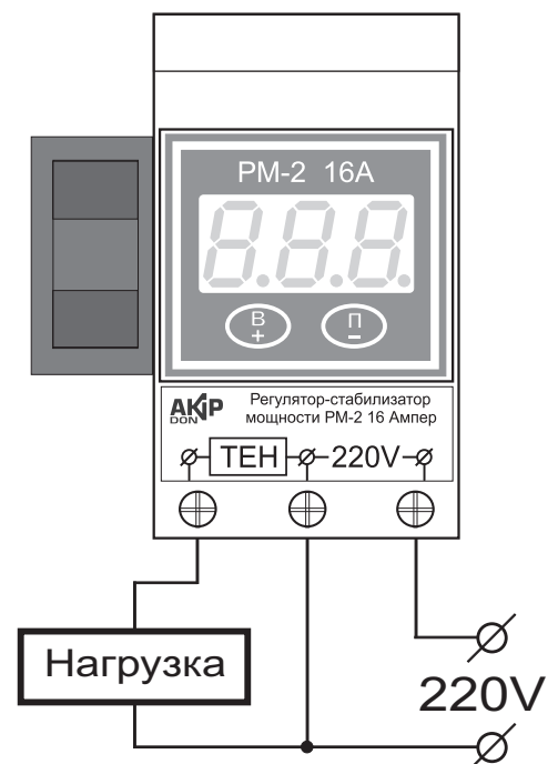
Рис. 1. Схема монтажа прибора.
