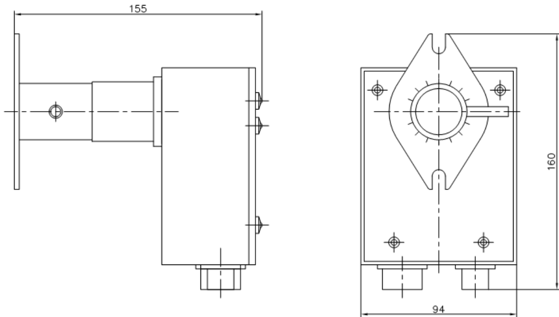
Габаритный чертёж фотодатчика ФДС-03-2К (в сборе с фланцем)
