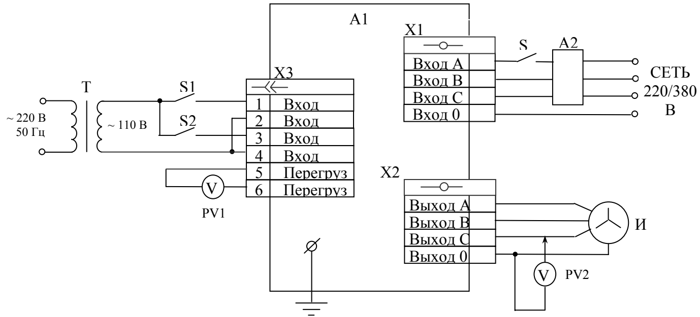
Схема электрическая подключения усилителя при проверке
