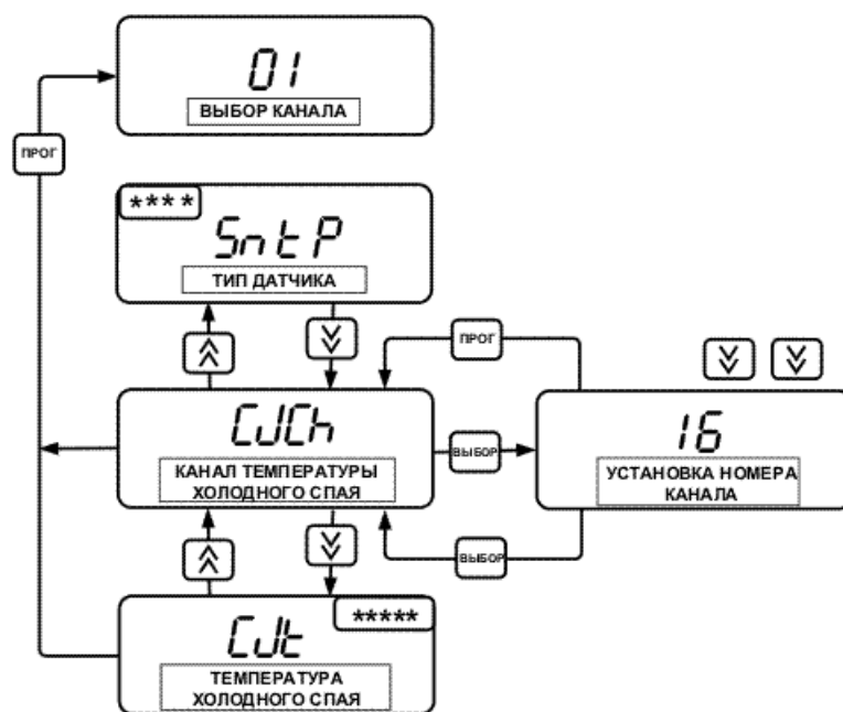
Рисунок 34 Применение термопар
