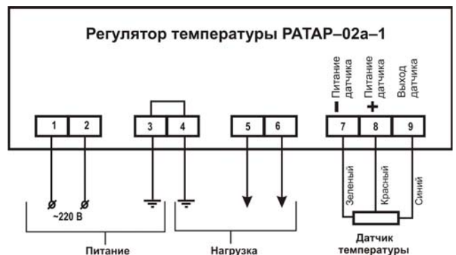
Схема электрическая подключения регулятора температуры РАТАР-02а-1
