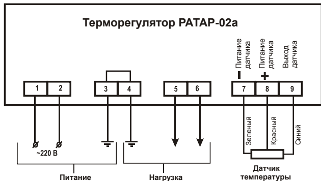
Схема электрическая подключения регулятора температуры РАТАР–02а
