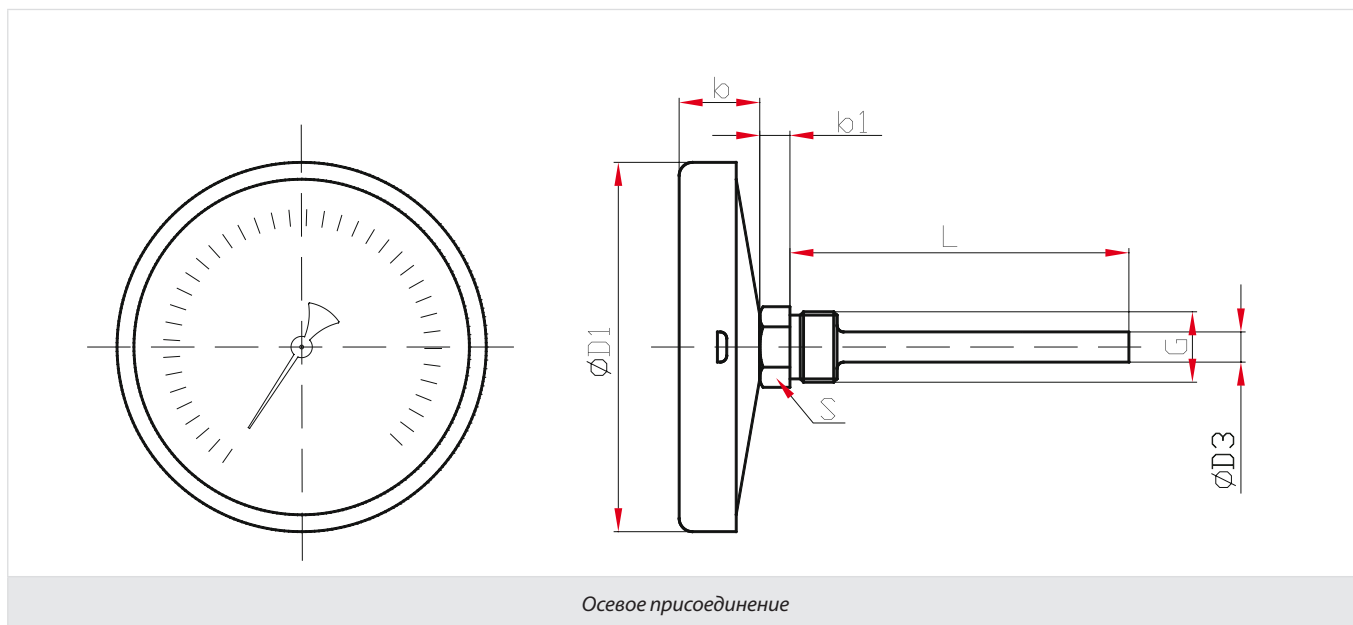
Основные размеры (мм), вес (кг)
