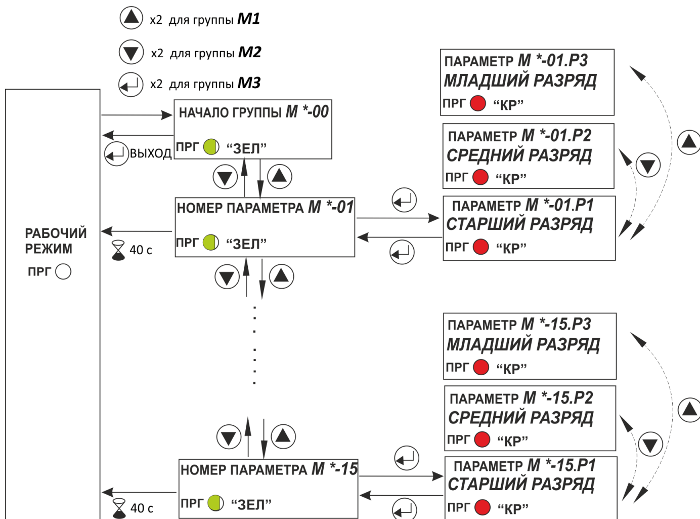
Рисунок 12 –Схема работы режима индикации параметров
