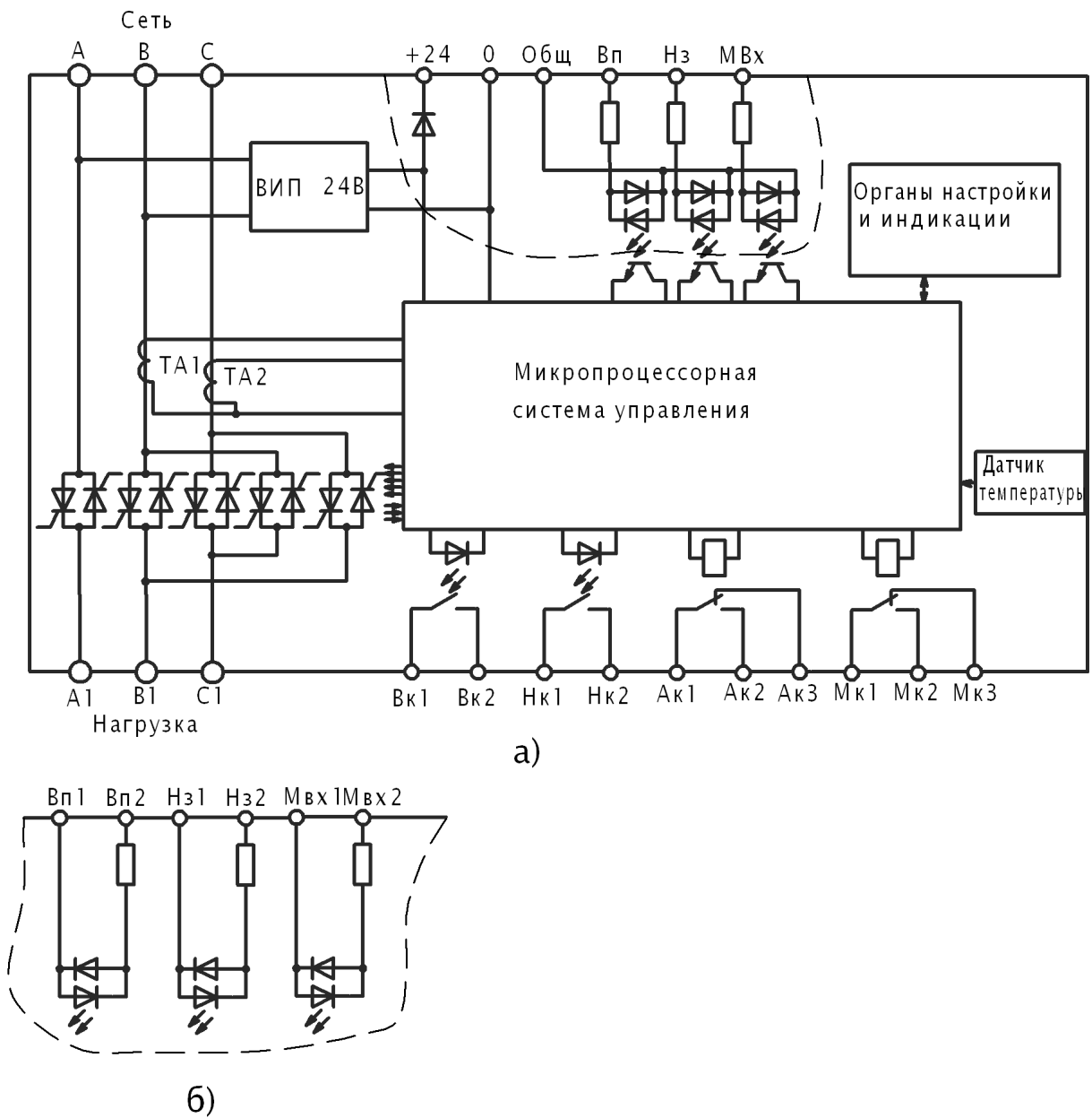
Рисунок 1 – Функциональная схема пускателя а) БСТ-ххР/380-3х б) схема входов управления для БСТ-ххР/380-0х и БСТ-ххР/380-2х
