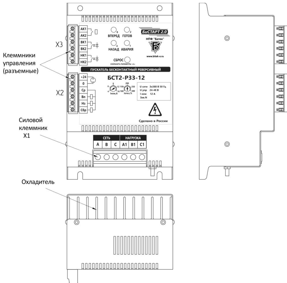
Рисунок 1 - Внешний вид пускателя БСТ2-Р33-12 (см. также Приложение А)
