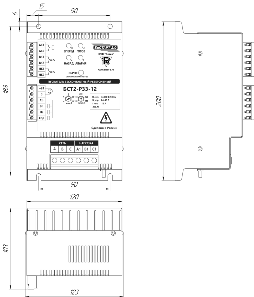
Рисунок А.1 – Габаритно-установочные размеры БСТ2-...-12
