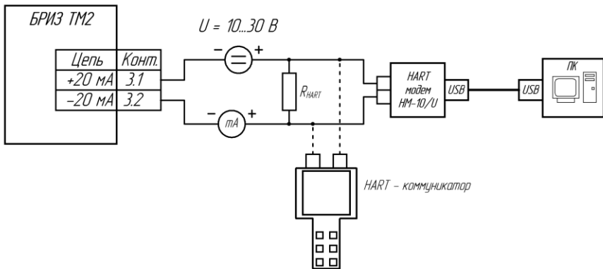
Рисунок А.8 – Схема электрическая подключений HART-коммуникатора и HART-модема к цепям пассивного аналогового выхода 4-20 мА БРИЗ TM2-Ex для обмена данными по HART-протоколу ( R_{HART} = 250...600 \text{ Ом} )
