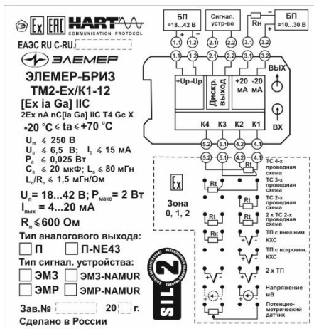
Рисунок Б.1 – Таблички с маркировкой
