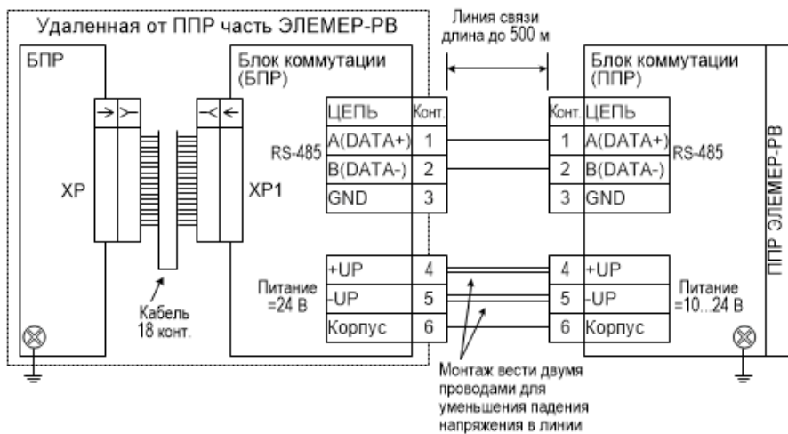
Рисунок А.11 – Схема подключений блока коммутации ЭЛЕМЕР-РВ (раздельное исполнение)
