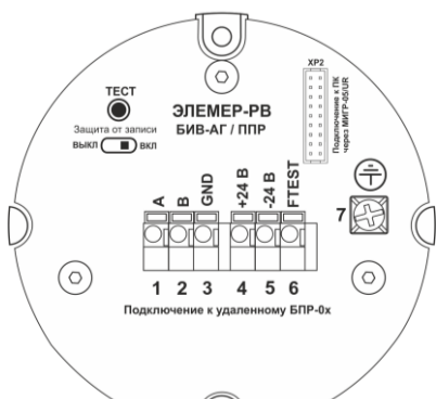
Блок коммутации (ППР)
