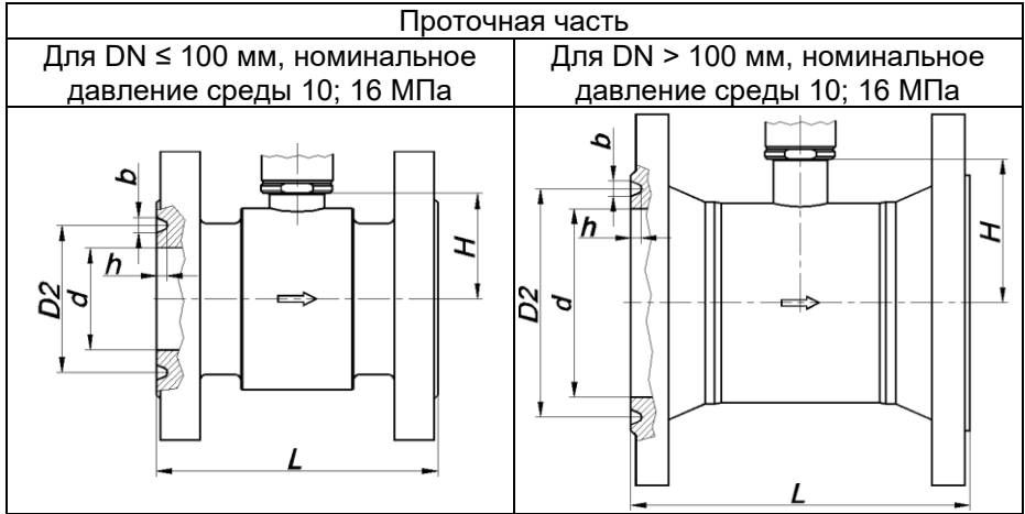
Рисунок Б.11 – Проточная часть расходомера (тип присоединения к процессу «фланцевый»)
