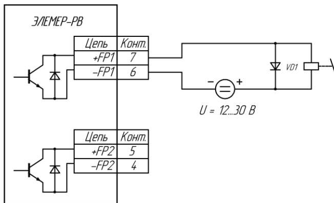
Рисунок А.8 – Схема электрическая подключений электромеханического исполнительного устройства к дискретным выходам ЭЛЕМЕР-РВ для режима дискретного выхода «Релейный».
