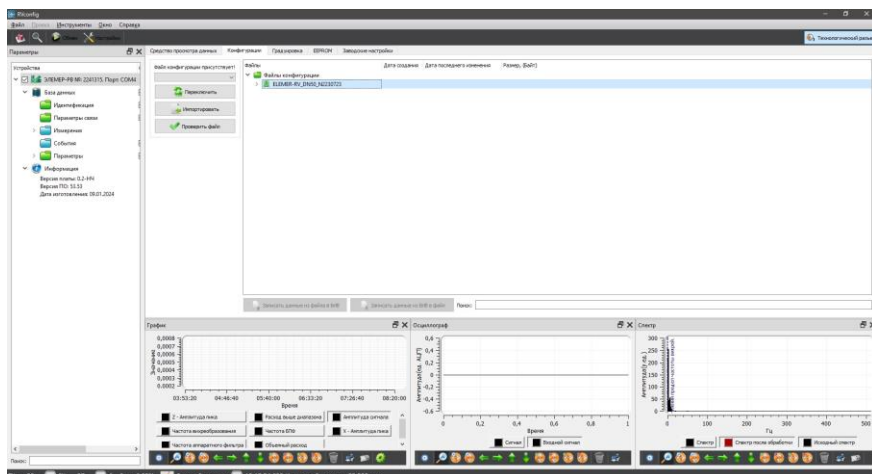
Рисунок 2.11 – Окно «Конфигурации»
