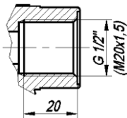
Рисунок Б.16 – Чертеж средств взрывозащиты (компактное исполнение, тип присоединения к процессу «зондовый с лубрикаторм»)»
