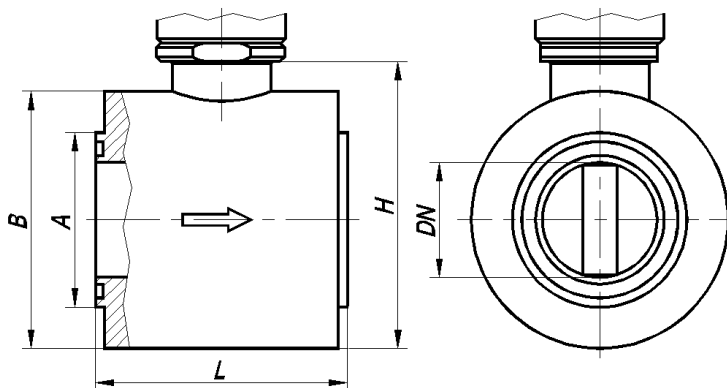
Рисунок Б.6 – Проточная часть расходомера (тип присоединения к процессу «сэндвич», тип 1, номинальное давление среды 2,5; 4,0; 6,3; 10,0; 16,0 МПа)
