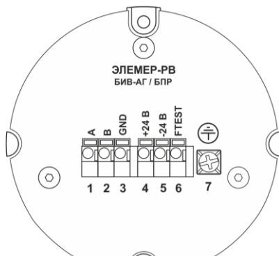
Блок коммутации (БПР)
