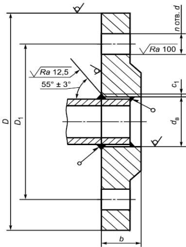
Тип фланца 01
