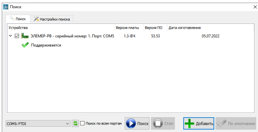
Рисунок 2.9 – Окно «Поиск»
