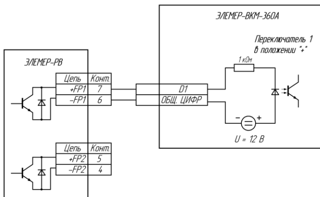
Рисунок А.9 – Схема электрическая подключений вычислителя расхода универсального «ЭЛЕМЕР-ВКМ-360» к дискретным выходам ЭЛЕМЕР-РВ. R_H = 1 \text{ кОм} .
