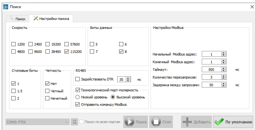
Рисунок 2.8 – Окно «Настройки поиска»
