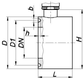
Рисунок Б.7 – Проточная часть расходомера (тип присоединения к процессу «сэндвич», номинальное давление среды 10; 16; 20 МПа)
