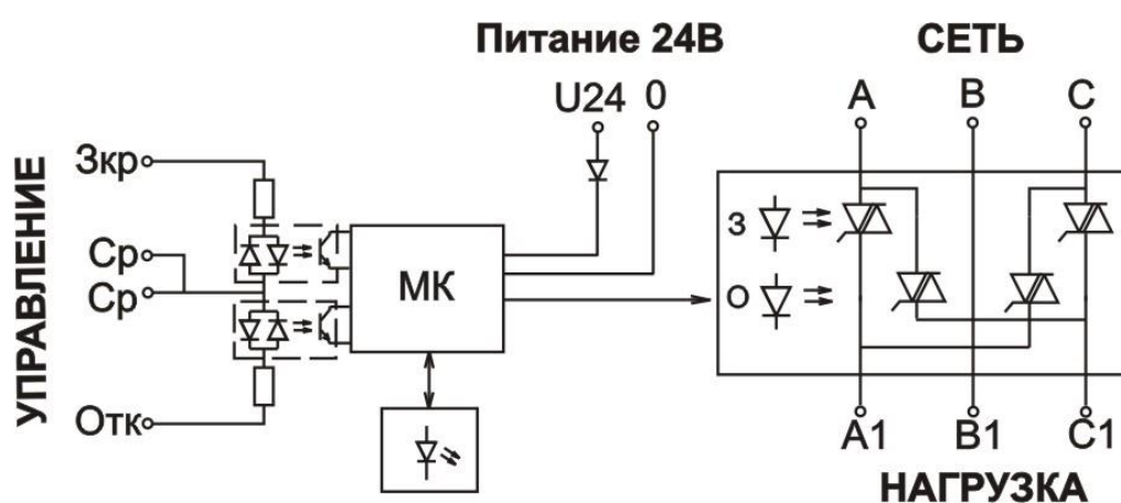
Рисунок 1 – Функциональная схема пускателей МСТ-300Р и МСТ-301Р
