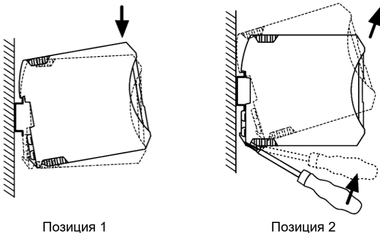
Рисунок 3.4 – Монтаж УЗИП (в корпусе ME MAX 12,5)
