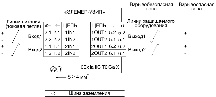
Рисунок Б.11 – Схема электрическая подключений «ЭЛЕМЕР-УЗИП-Ex» (тип корпуса ME MAX 12,5)
