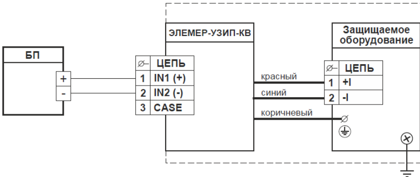
Рисунок Б.8 – Схема электрических подключений «ЭЛЕМЕР-УЗИП» (тип корпуса KB)
