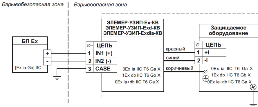
Рисунок Б.9 – Схема электрических подключений «ЭЛЕМЕР-УЗИП-Ex», «ЭЛЕМЕР-УЗИП-Exd», «ЭЛЕМЕР-УЗИП-Exdia» (тип корпуса KB)
